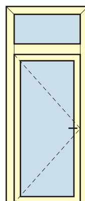
Enkele binnen-draaiende deur met vast bovenlicht
