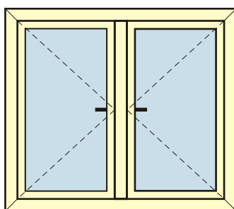
Dubbel opendraaiend raam met T-stijl (OD-OD)
